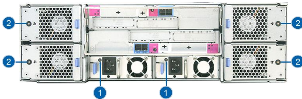
图 3-26 3U 扩展柜电源、风扇指示灯
