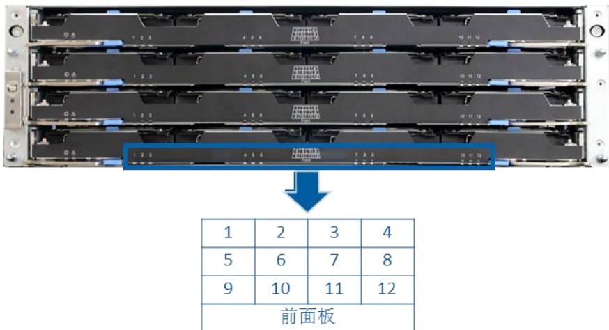
图 2-18 3U 机柜硬盘序号对应关系
