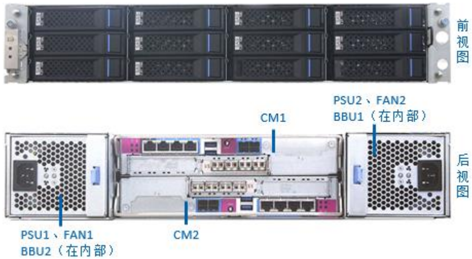
图 2-1 2U12 盘位前面板和后面板视图
