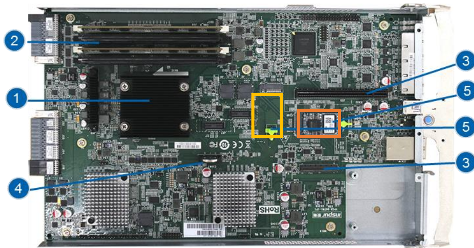
图 2-7 控制器内结构图
