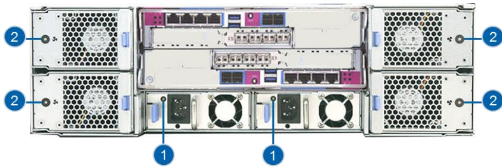
图 2-21 3U 机柜电源风扇指示灯
