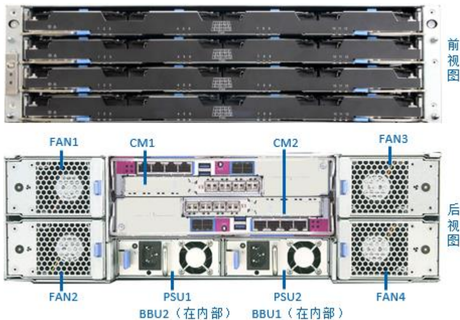
图 2-3 3U48 盘位前面板和后面板视图
