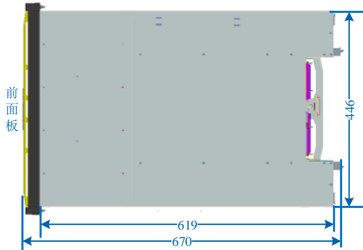
图 2-5 2U 控制柜尺寸
