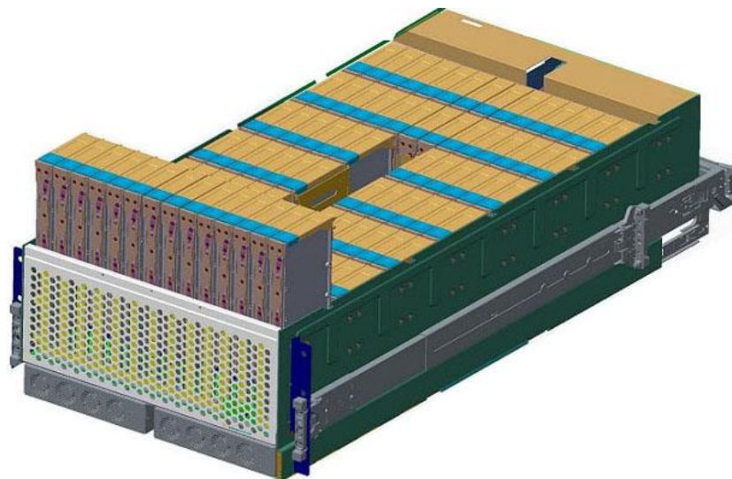
图 3-6 5U 硬盘模块结构图
