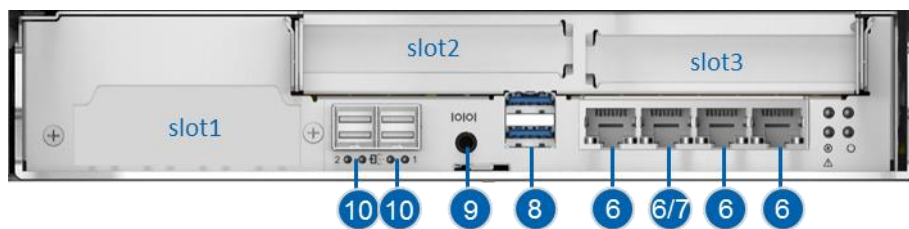
图 2-8 控制器后视图
