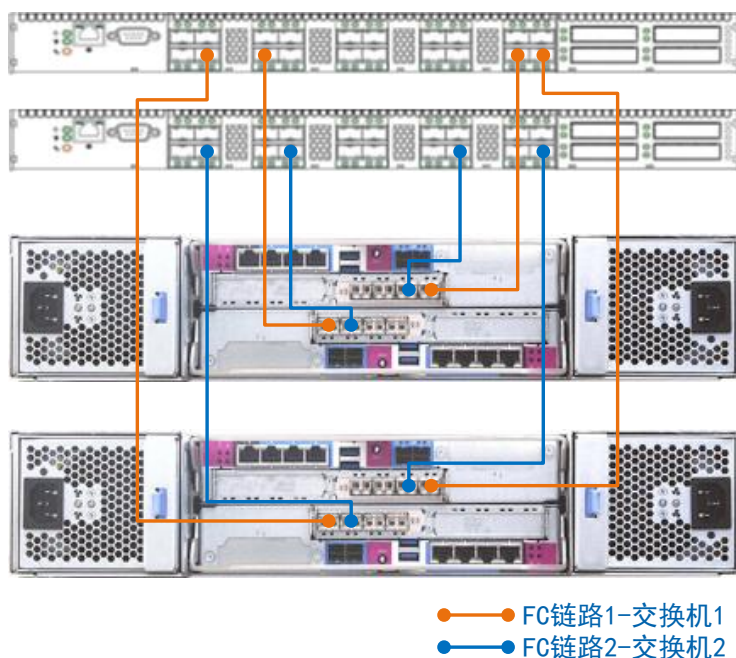
图 4-1 四个控制器（2 个控制柜）冗余连接方式-AS2600G2
