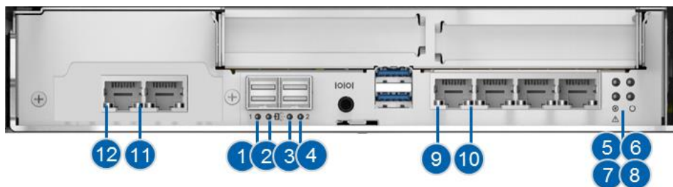
图 2-19 控制柜后面板指示灯
