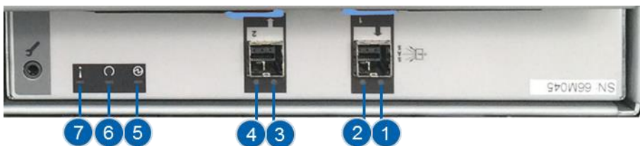
图 3-24 5U 硬盘扩展柜 ESM 后端指示灯
