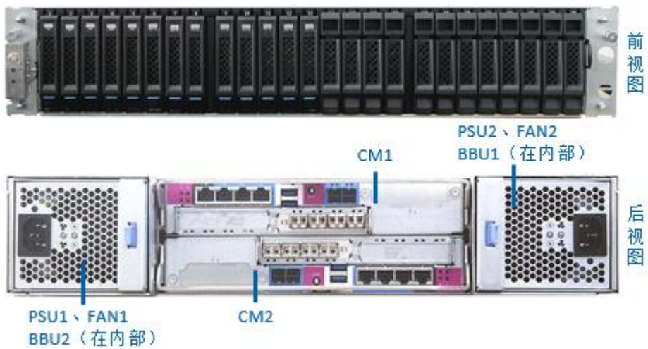
图 2-2 2U25 盘位前面板和后面板视图
