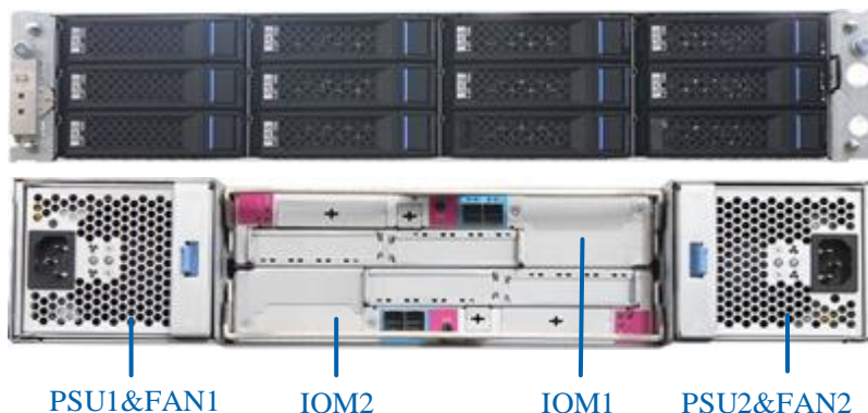
图 3-1 2U12 盘位前面板和后面板视图
