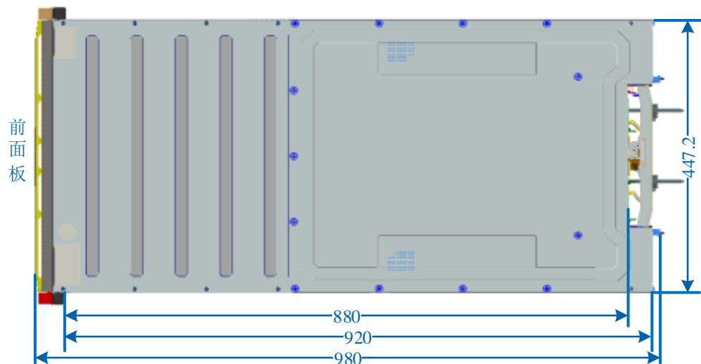
图 2-6 3U 控制柜尺寸
